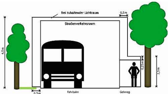
(Grafik: Landratsamt Bayreuth – Straßenlichtraumprofil, das von Bewuchs freizuhalten ist)
